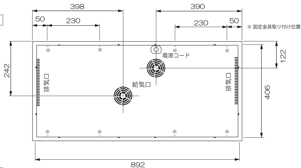
背面図
