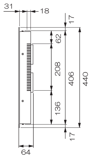
右側面図
