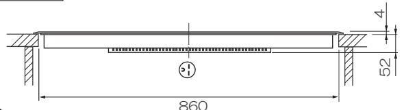
正面図
