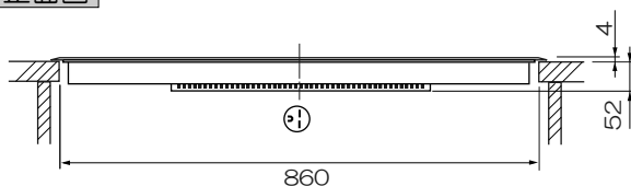
正面図
